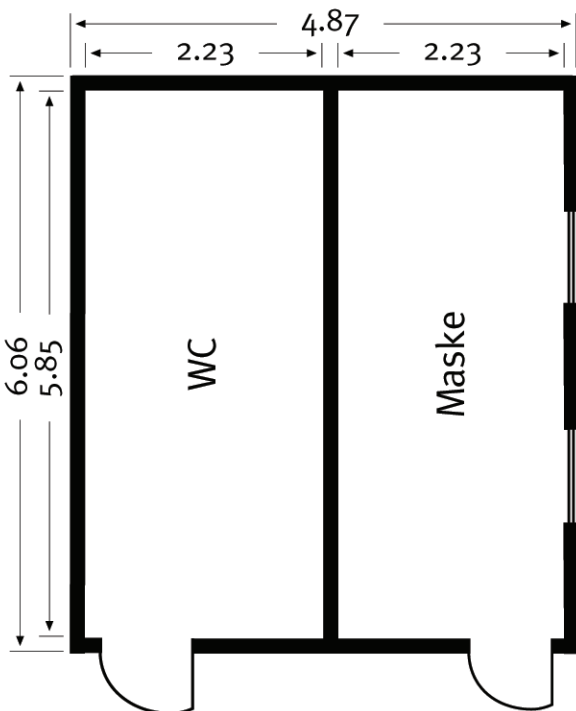
Grundriß EG.
